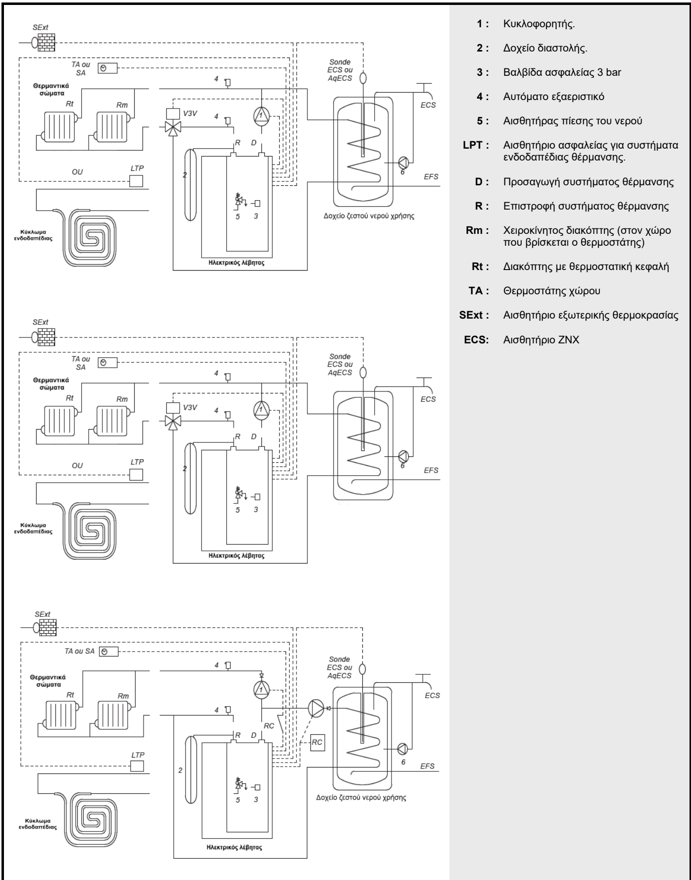
Σχήμα 7: Σύνδεση ηλεκτρικού λέβητα Gialix MA με σύστημα θέρμανσης.
