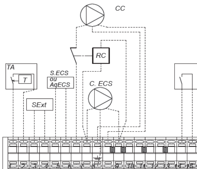
Σχήμα 8: Ηλεκτρική συνδεσμολογία εξωτερικών οργάνων και αισθητήριων.
