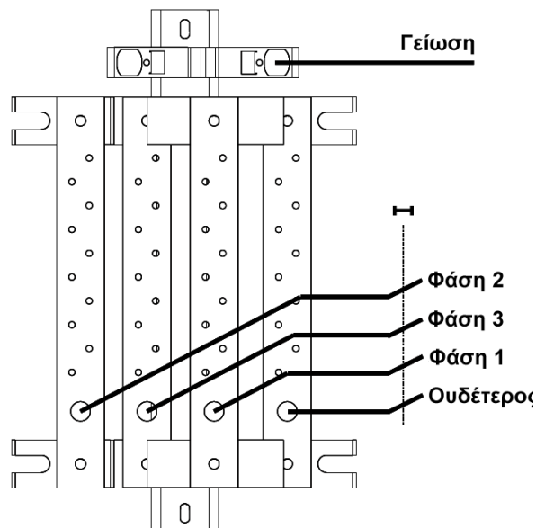
Συνδεσμολογία κεντρικής παροχής
