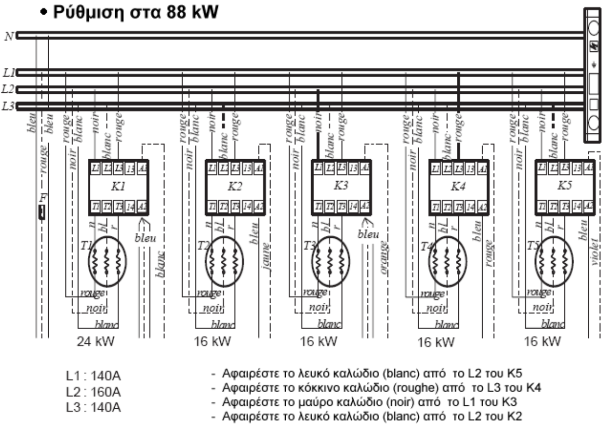
Σχήμα 16: Μεταβολή της ισχύος του λέβητα Gialix 120MA με αφαίρεση καλωδίων.
