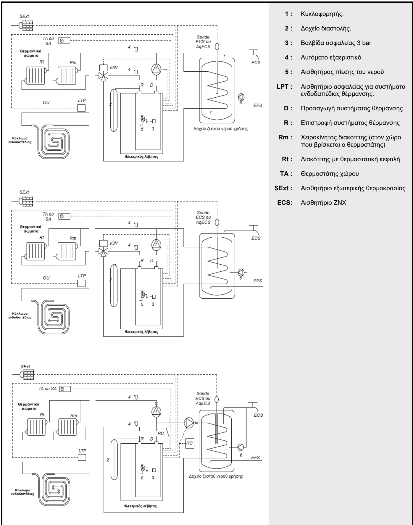
Σχήμα 7: Σύνδεση ηλεκτρικού λέβητα Gialix με το σύστημα θέρμανσης και ζεστού νερού χρήσης
