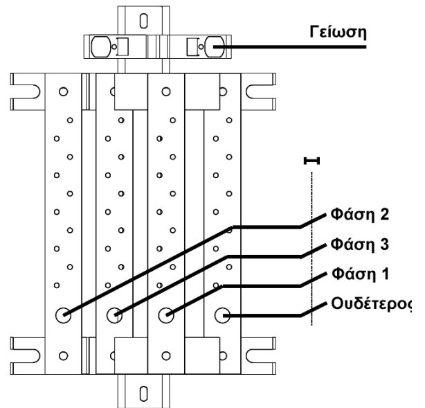
Συνδεσμολογία κεντρικής παροχής
