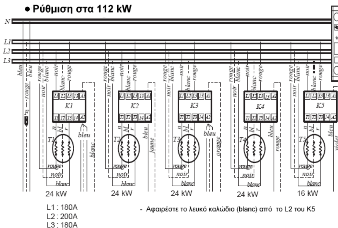
Σχήμα 13: Μεταβολή της ισχύος του λέβητα Gialix 120MA με αφαίρεση καλωδίων.
