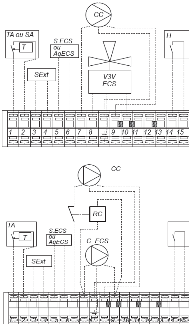
Σχήμα 8: Ηλεκτρική συνδεσμολογία εξωτερικών οργάνων και αισθητήριων.
