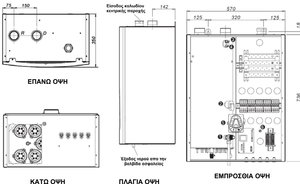
Σχήμα 2 : Βασικές διαστάσεις λέβητας Gialix 120Kw.
