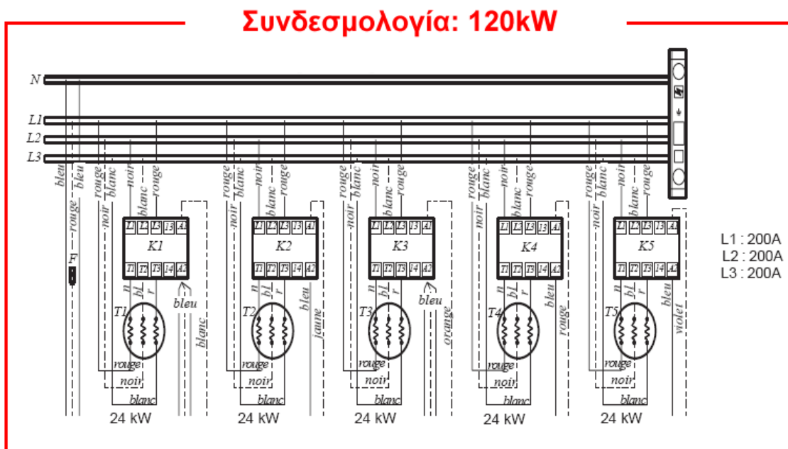
Σχήμα 12: Εργοστασιακή συνδεσμολογία λέβητα Gialix 120MA
