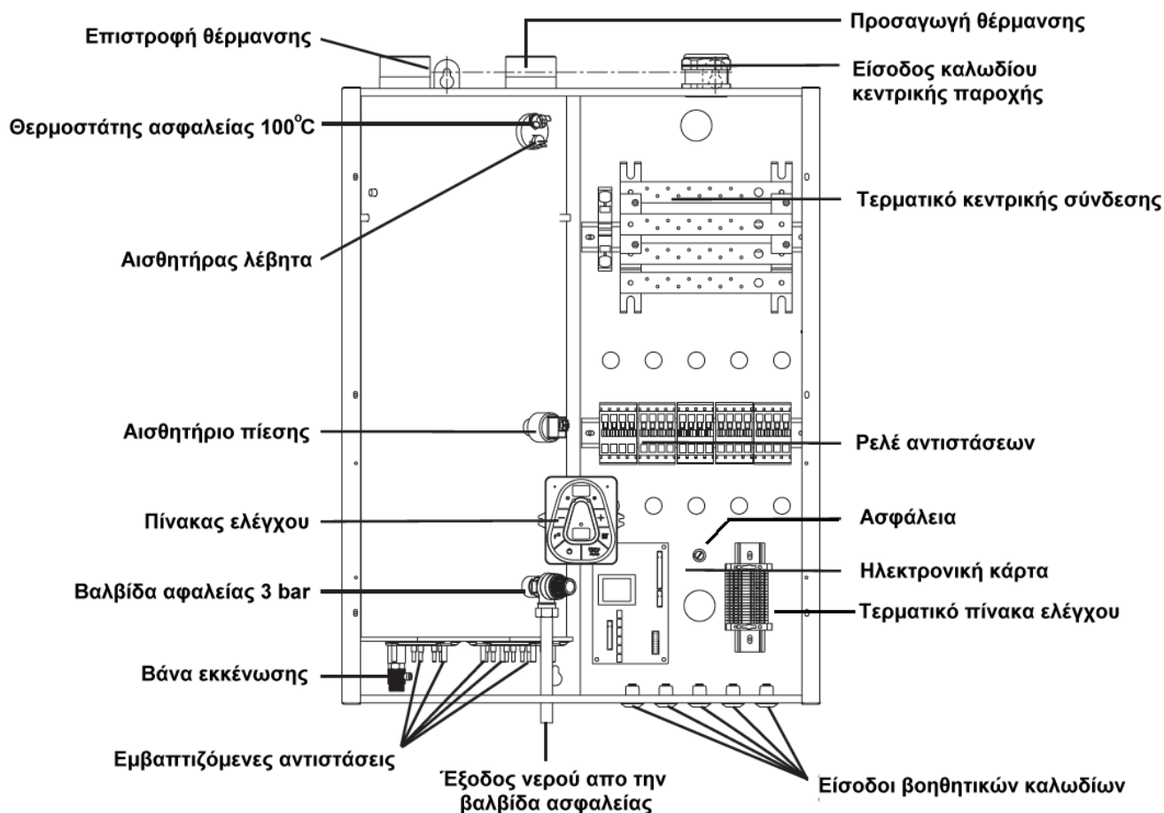
Σχήμα 1 : Λέβητας Gialix 120kW.
