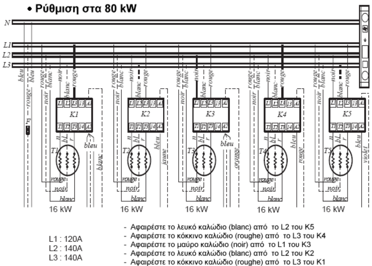
Σχήμα 17: Μεταβολή της ισχύος του λέβητα Gialix 120MA με αφαίρεση καλωδίων.
