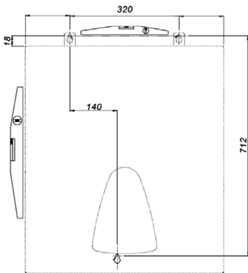
Σχήμα 3: Στήριξη λέβητα στον τοίχο
